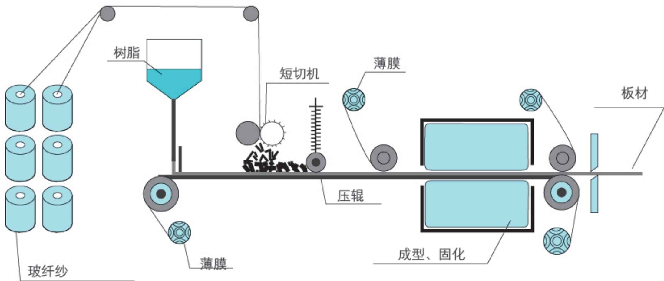
连续板材成型示意图
